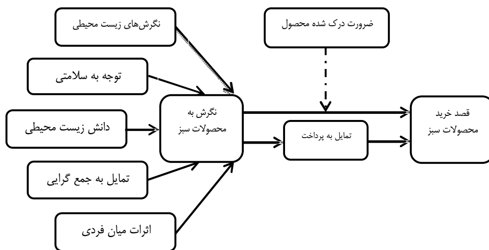
شکل ۱: مدل مفهومی تحقیق (منابع: لاروچه و همکاران (۲۰۰۱)، مصطفی (۲۰۰۷)، آریال و همکاران (۲۰۰۹)، چن (۲۰۰۹)، چیا و فائو (۲۰۱۱)، لیزاواتی آمان و همکاران (۲۰۱۲)، کلس و بکیمبتوا (۲۰۱۳)، خویریا و سوامتارو (۲۰۱۳))
