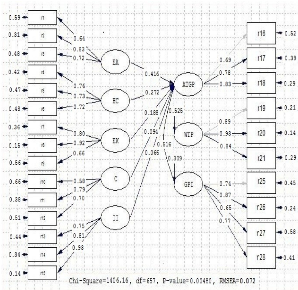
شکل (۲): مدل تحقیق در حالت تخمین ضرایب مسیر
